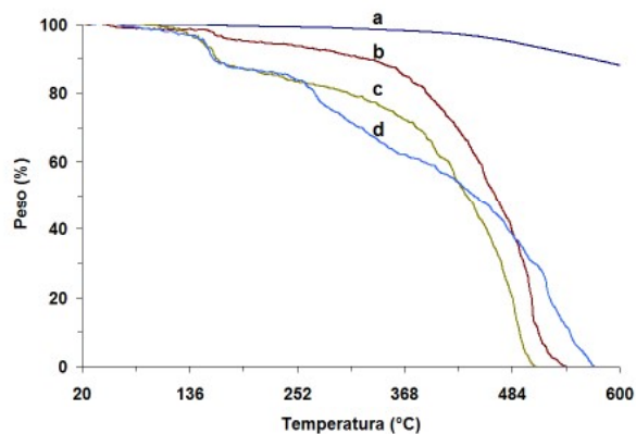
Fig. 5. Termogramas de PANi sintetizada por diferentes vías y condiciones de reacción. a) CPANi, b) BPANi a pHo = 1 en AcOH al 50% (v/v), c) BPANi a pHo = 0.15 en AcOH al 75% (v/v), d) EPANi.
