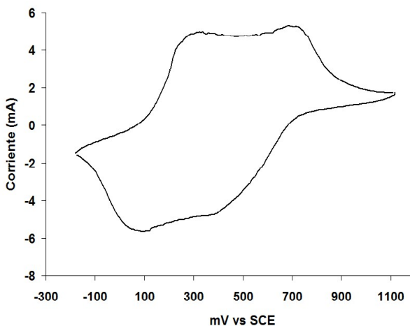
Fig. 7. Curva voltamétrica de la polianilina sintetizada biomiméticamente (BPANi).
